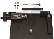
Grundgerät zur Zugfestigkeitsmessung Bestellnummer 1244045
