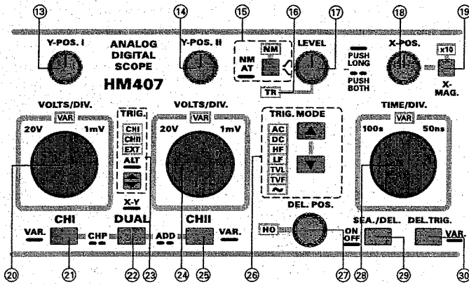
(29) SEA./DEL. - ON/OFF -Drucktaste mit zwei Funktionen.
