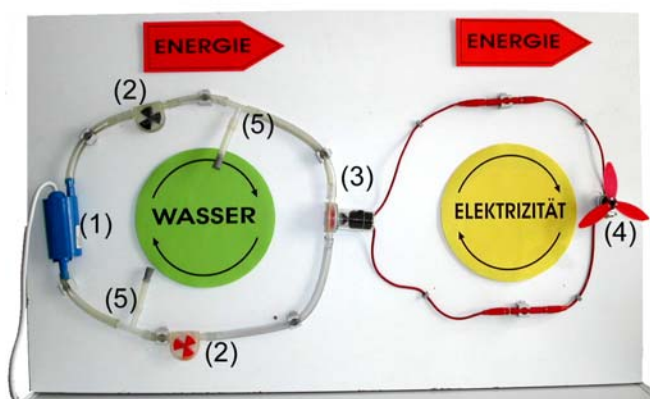
Abb. 2: hydraulischer Energie-Träger-Stromkreis
