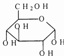
Fructose
