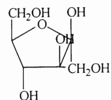
Saccharose
