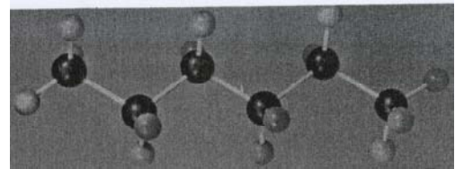
Hexan
