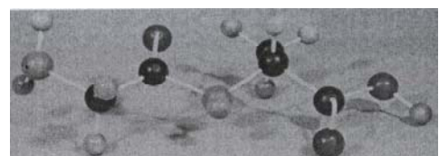
Dipeptid
