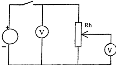
Aufbau Potentiometer
