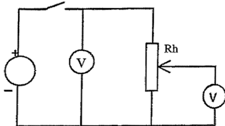
Aufbau Potentiometer
